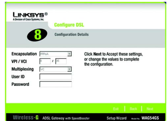
Figure 5-14 : Ecran Configure DSL - PPPoA (Configuration DSL - PPPoA) de l'Assistant de configuration
